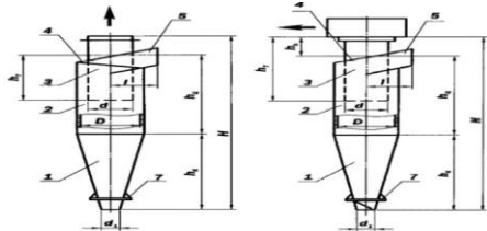
Циклон ЦН-11 без улитки
